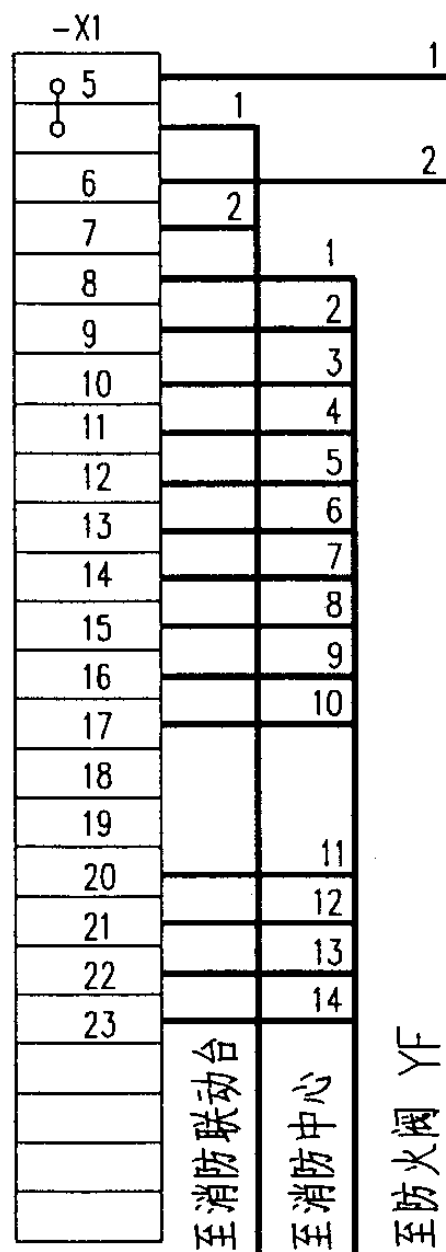
外部接线图
