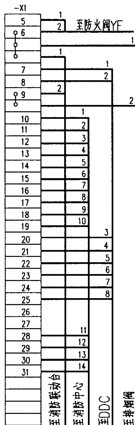
外部接线图
