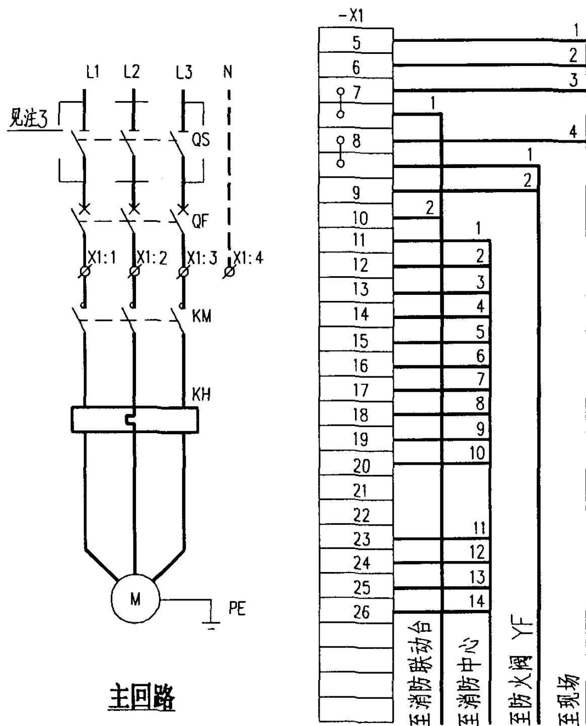
外部接线图
