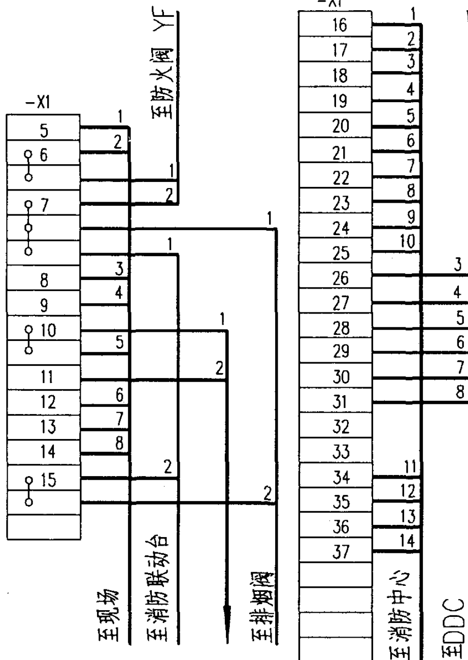
外部接线图
