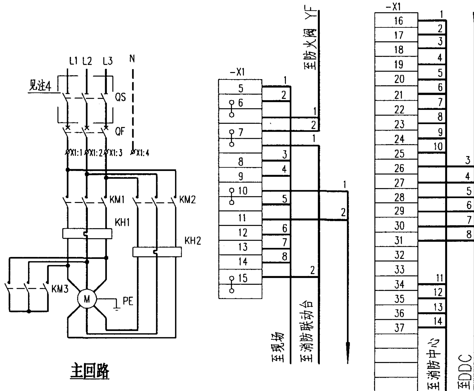
外部接线图
