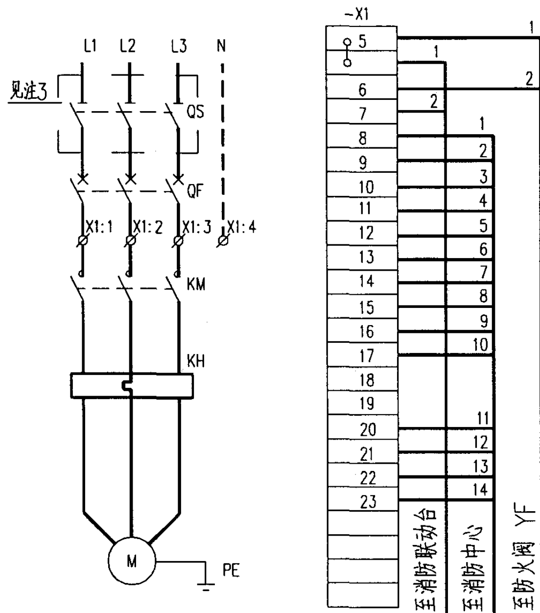
主回路
