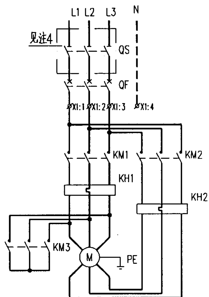
主回路
