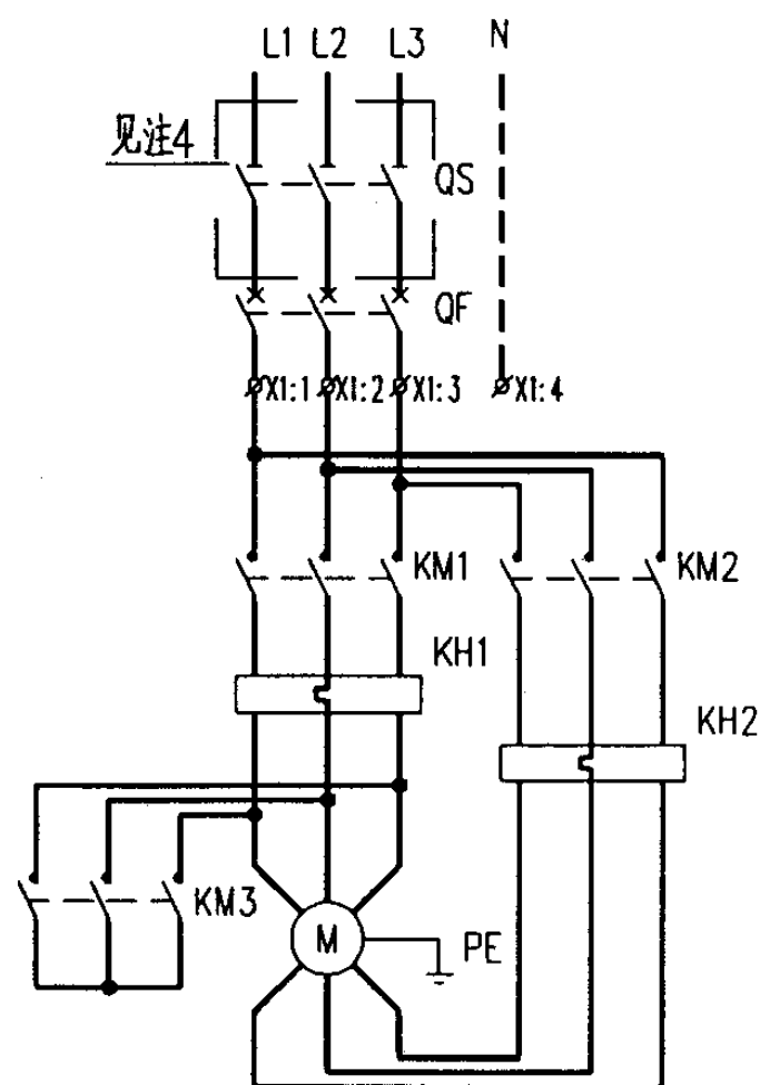
主回路
