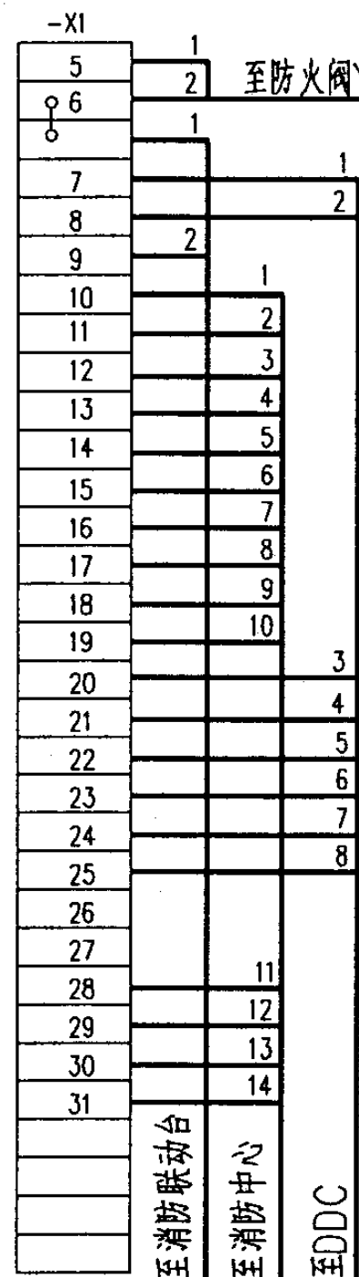
外部接线图
