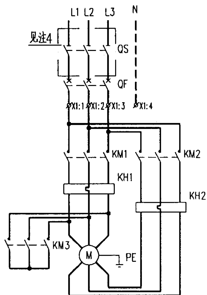
主回路
