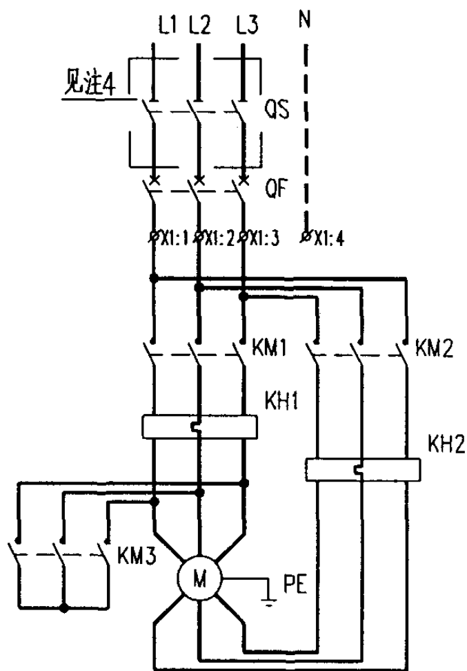
主回路
