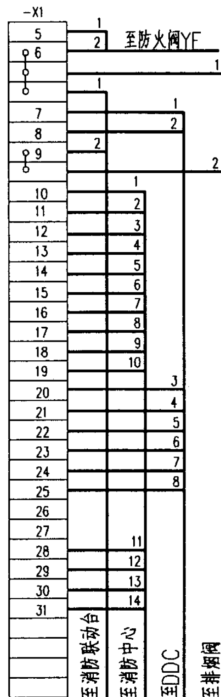
外部接线图
