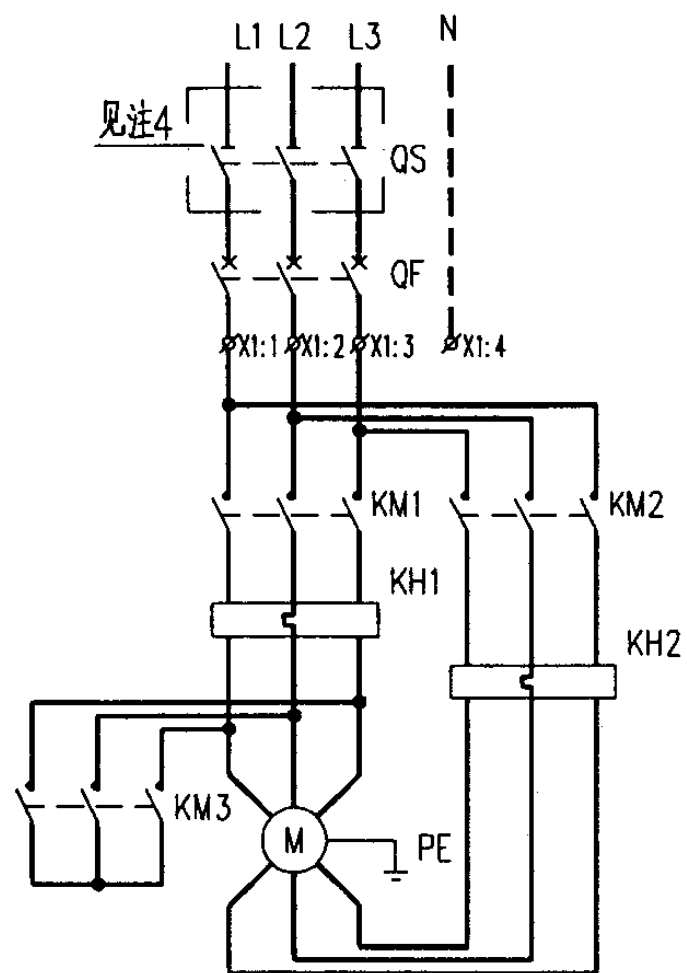
主回路
