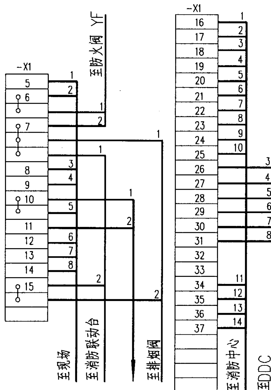
外部接线图
